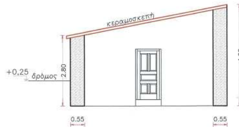
ΤΟΜΗ Γ - Γ' ΙΣΟΓΕΙΑΣ ΑΠΟΘΗΚΗΣ (ΜΕΤΑ ΤΗΝ ΕΠΙΣΚΕΤΗ)
