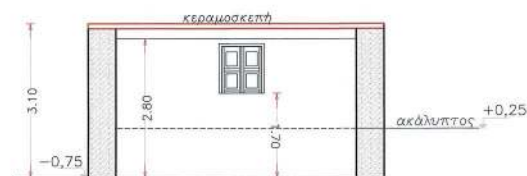
ΤΟΜΗ Δ - Δ' ΥΦΙΣΤΑΜΕΝΗΣ ΑΠΟΘΗΚΗΣ (ΜΕΤΑ ΤΗΝ ΕΠΙΣΚΕΤΗ)
