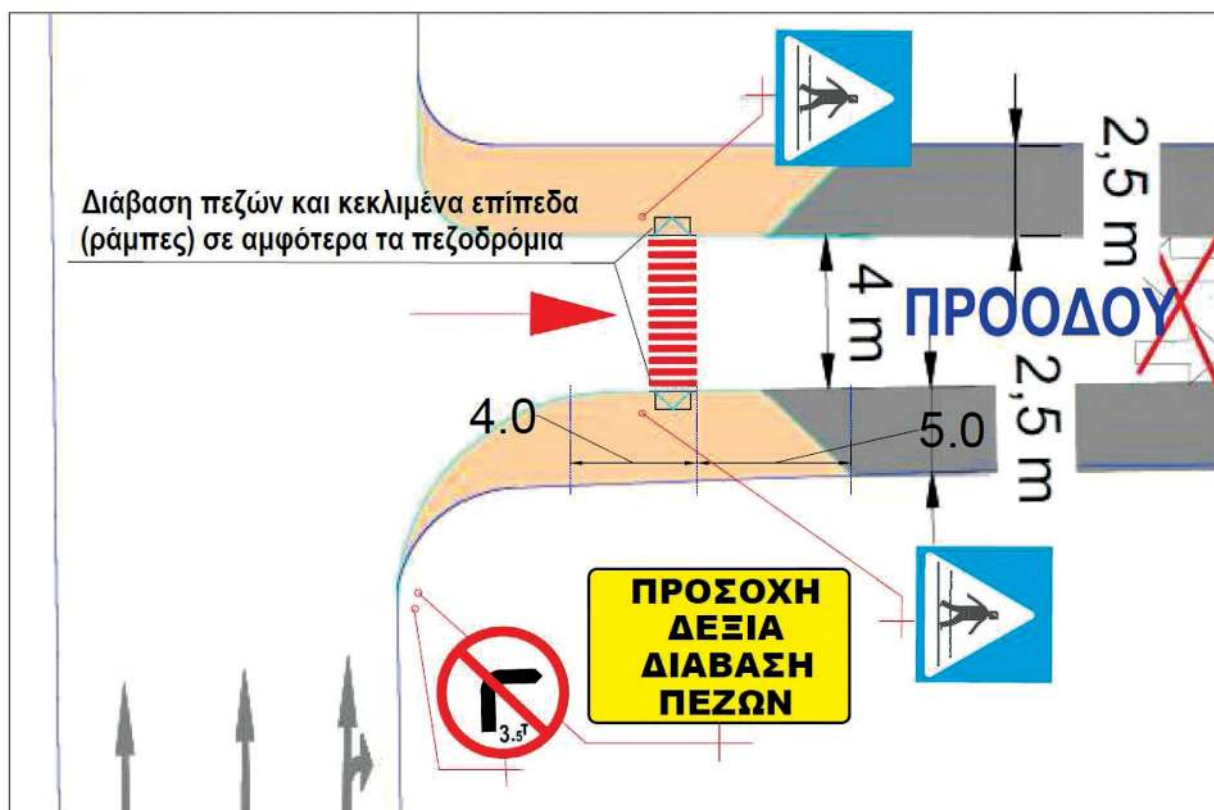
Εικόνα 1: Ενδεικτική σκαριφηματική απεικόνιση προτεινόμενων παρεμβάσεων επί της οδού ΠΡΟΟΔΟΥ.
