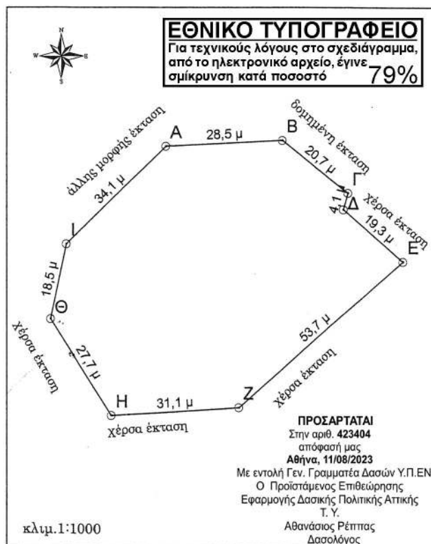
ΤΟΠΟΓΡΑΦΙΚΟ ΔΙΑΓΡΑΜΜΑ
