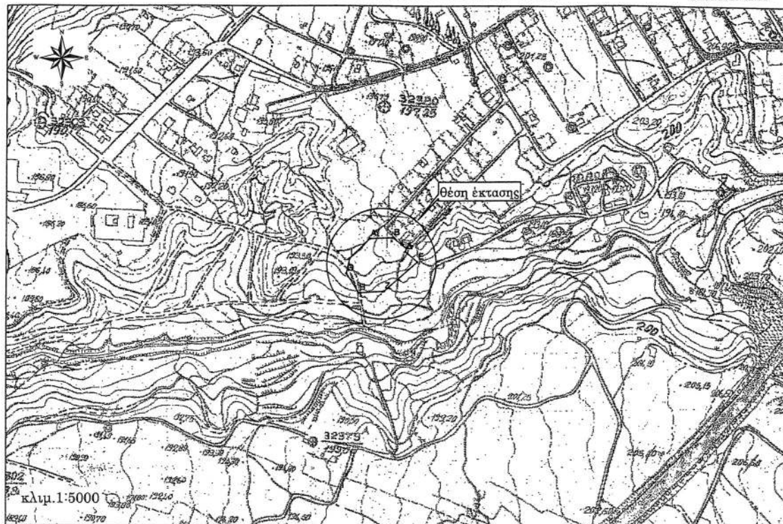
ΤΟΠΟΓΡΑΦΙΚΟ ΔΙΑΓΡΑΜΜΑ
