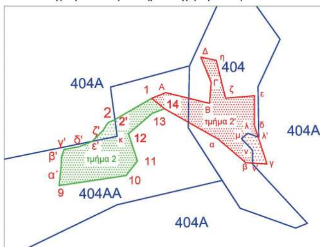
Ανάπτυγμα με απόσ/μα Κτημ./κου χάρτη σε κλίμακα 1:1500
