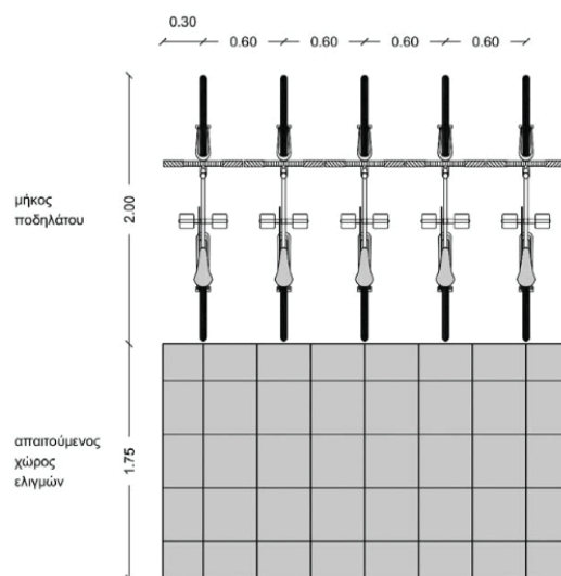
Σχήμα 1: διάταξη θέσεων σε σειρά
