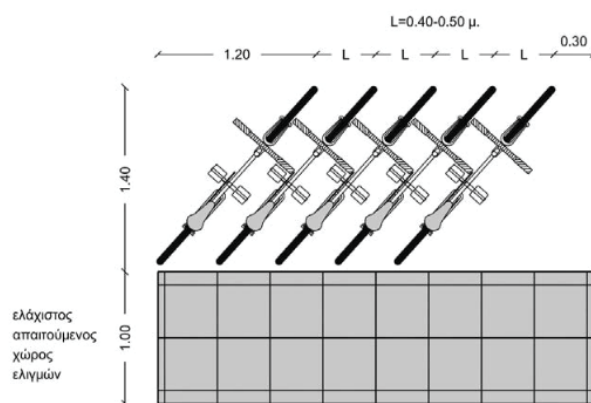
Σχήμα 2: διάταξη θέσεων υπό γωνία σε σειρά
