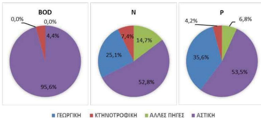
Σχήμα 5-6. Κατανομή ετήσιων ρυπαντικών φορτίων BOD, N και P στα ΕΥΣ και ΥΥΣ από διάχυτες πιέσεις στη ΛΑΠ Πάμισου - Νέδοντος - Νέδας (EL0132)
