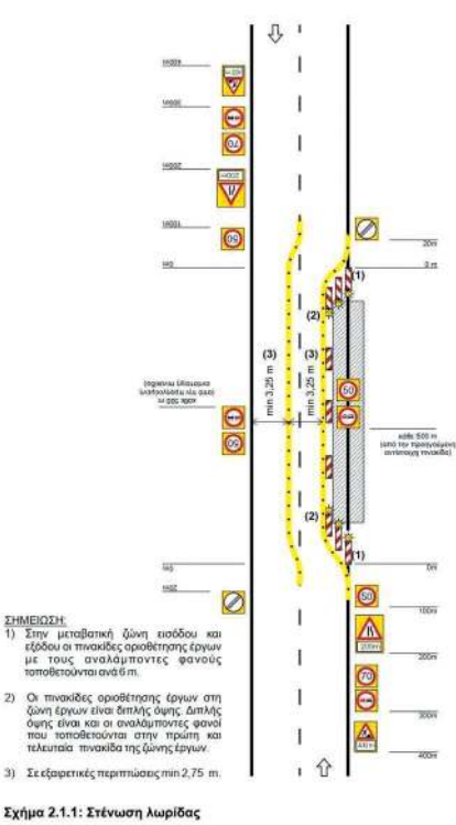
Σχήμα 2.1.1: Στένωση λωρίδας
