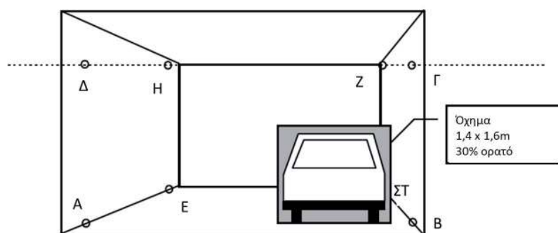
Εικόνα 13: Γενικευμένο σχέδιο εφαρμογής μεθόδου LTP με εμπόδιο όχημα (παράδειγμα).
