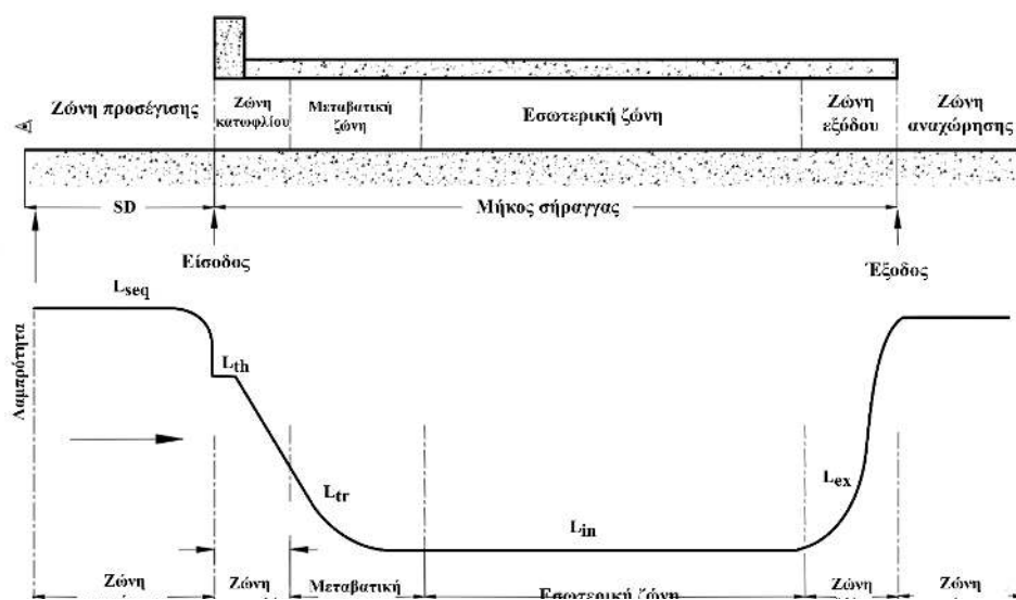
Εικόνα 17: Ζώνες φωτισμού σήραγγας και τυπική διακύμανση λαμπρότητας οδοστρώματος.
