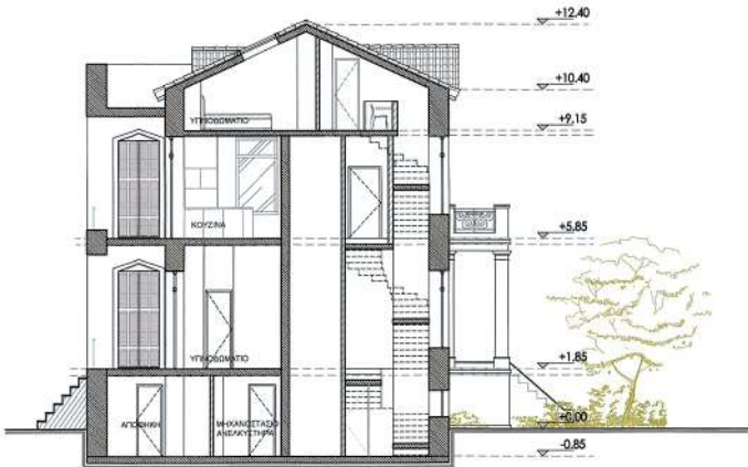
ΤΟΜΗ Β-Β
