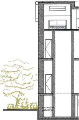
ΤΟΜΗ Γ-Γ
