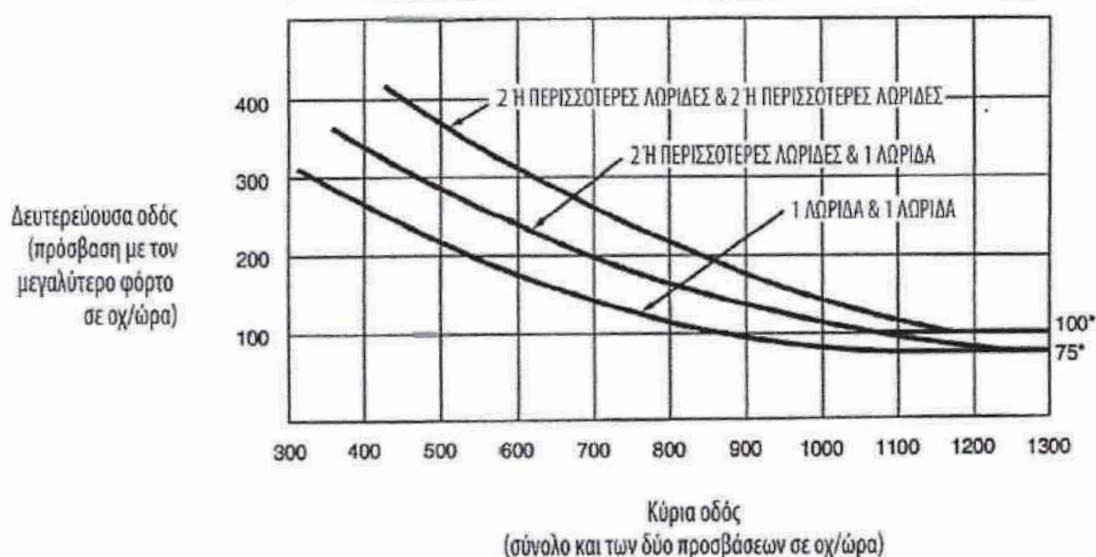
Γράφημα 3.2. Κριτήριο 3, Ώρα Αιχμής (Συντελεστής 70%)
