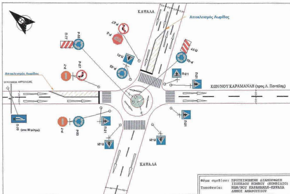
Σχέδιο 1: Προτεινόμενη διαμόρφωση κυκλικού κόμβου Κων. Καραμανλή και Ασπ. Καψάλα
