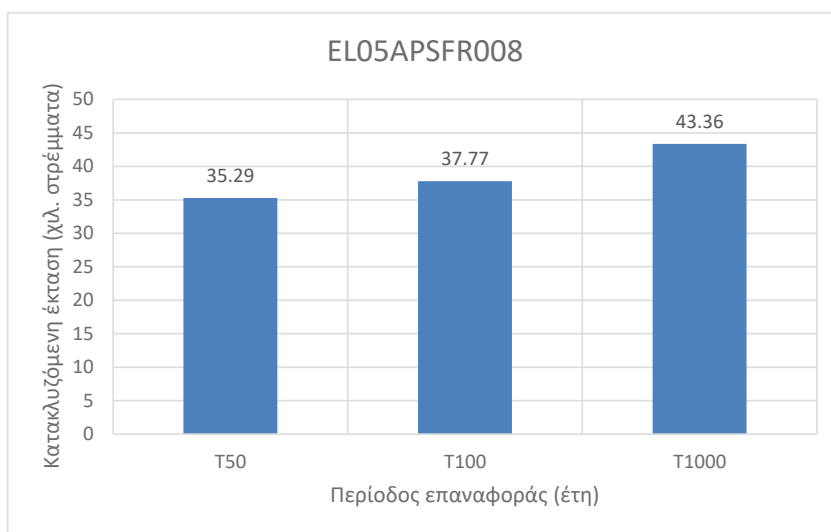
Εικόνα 3-32 Κατακλυζόμενες εκτάσεις για τις πλημμύρες περιόδου επαναφοράς 50, 100 και 1.000 ετών καθώς και για τις θαλάσσιες πλημμύρες περιόδου επαναφοράς 50 και 100 ετών στη EL05APSFR008
