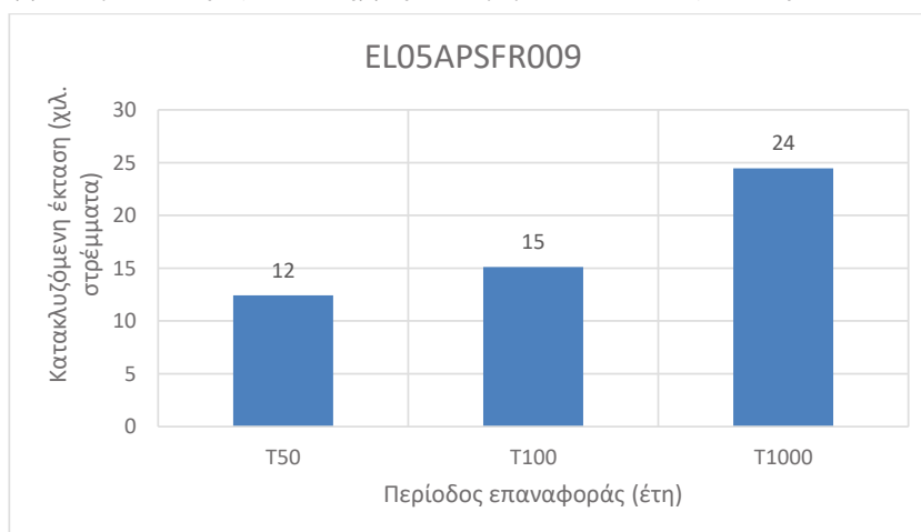
Εικόνα 3-34 Κατακλυζόμενες εκτάσεις για τις πλημμύρες περιόδου επαναφοράς 50, 100 και 1.000 ετών στη EL05APSFR009
