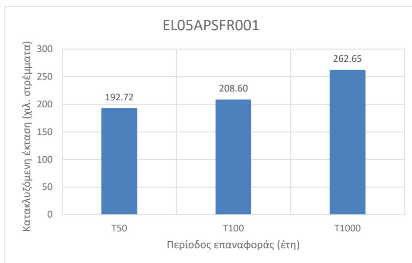
Εικόνα 3-21 Κατακλυζόμενες εκτάσεις στη EL05APSF001 για τις πλημμύρες περιόδου επαναφοράς 50, 100 και 1 000 ετών
