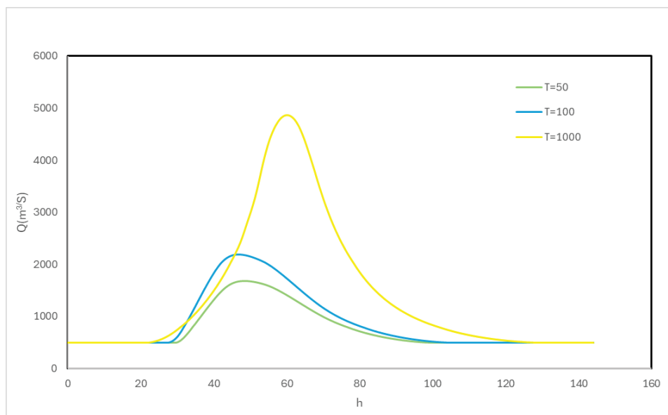
Πλημμυρογράφημα Εξόδου π. Αράχθου κατάντη ταμιευτήρα Πουρναρίου (μέσες συνθήκες)
