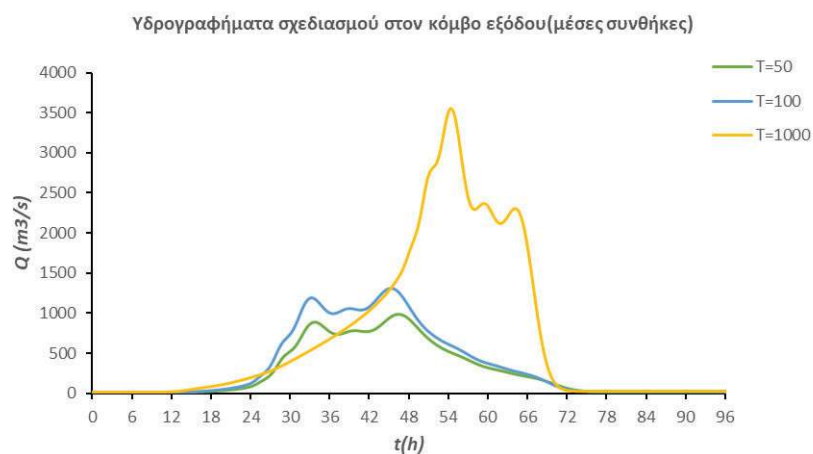
Εικόνα 3-19 Πλημμυρογραφήματα Εξόδου για τις μέσες συνθήκες των σημαντικότερων ποταμών του ΥΔ Ηπείρου
