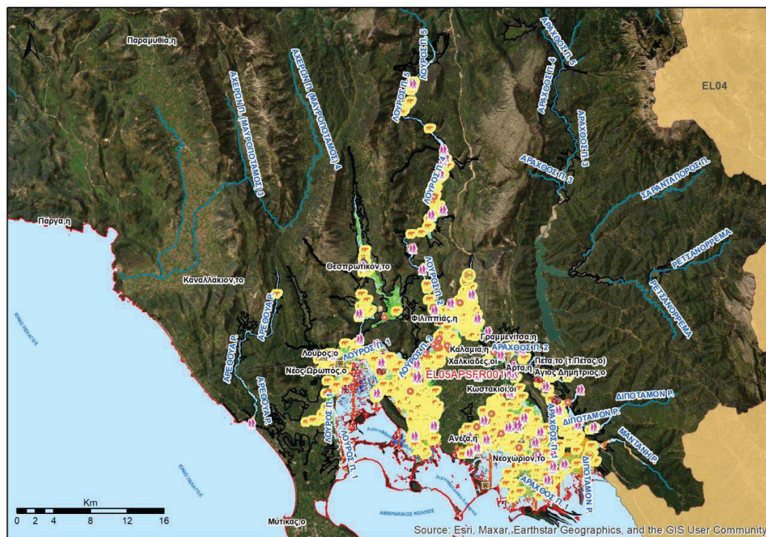
Εικόνα 3-55 Δυνητικά θιγόμενες χρήσεις γης, υποδομές και οικονομικές δραστηριότητες στη EL05APSFR001
