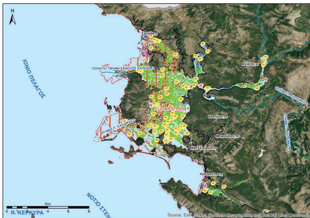
Εικόνα 3-60 Δυνητικά θιγόμενες χρήσεις γης, υποδομές και οικονομικές δραστηριότητες στη EL05APSFR008
