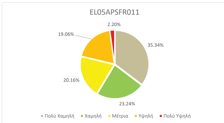
Εικόνα 3-94 Ποσοστό της συνολικής ζώνης κατάκλυσης ανά κατηγορία τρωτότητας για τη EL05APSFR011
