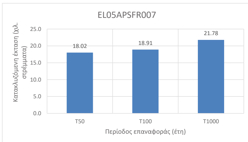
Εικόνα 3-30 Κατακλυζόμενες εκτάσεις για τις πλημμύρες περιόδου επαναφοράς 50, 100 και 1.000 ετών στη EL05APSR007
