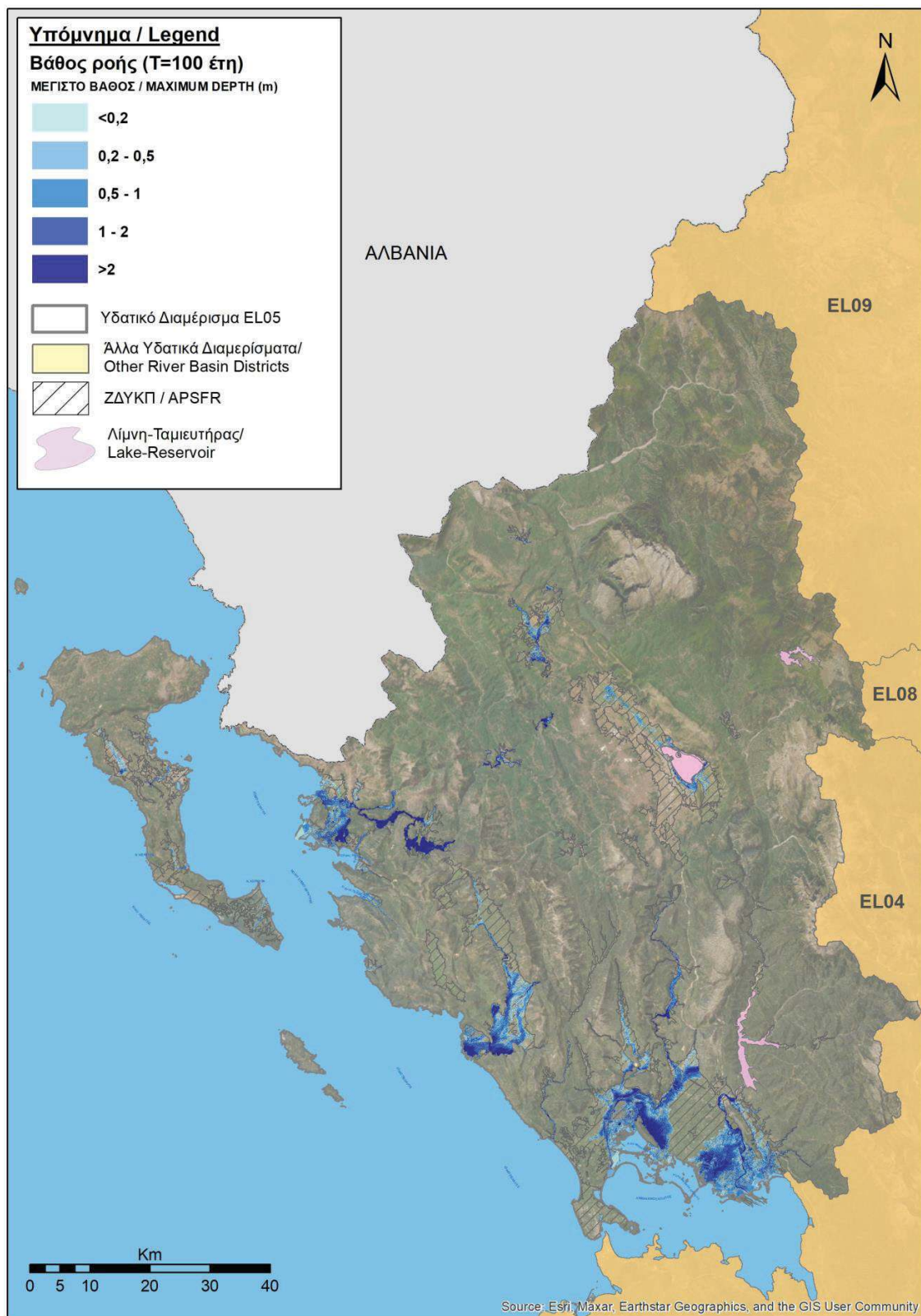
Εικόνα 3-46: Βάθος ροής και μέγιστο εύρος κατάκλυσης για πλημμύρα με περίοδο επαναφοράς T=100 έτη για το Υδατικό Διαμέρισμα Ηπείρου (EL05)
