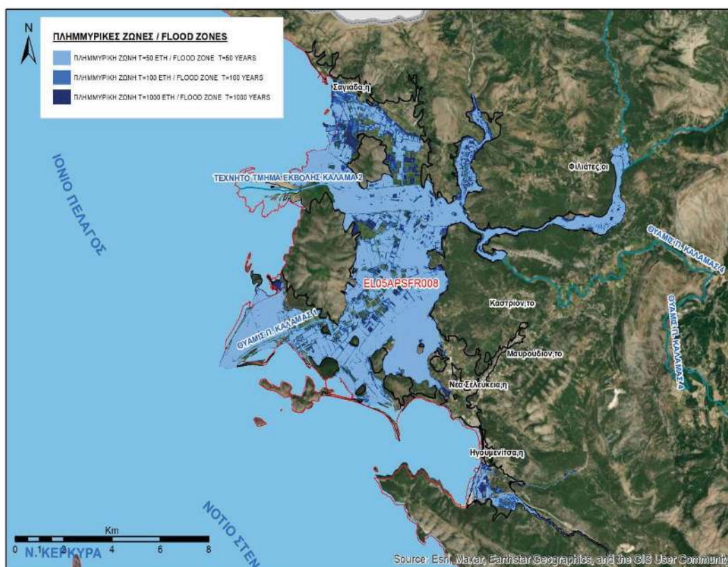
Εικόνα 3-33 Ζώνες κατάκλυσης για T=50, T=100 και T=1000 έτη για την EL05APSFR008
