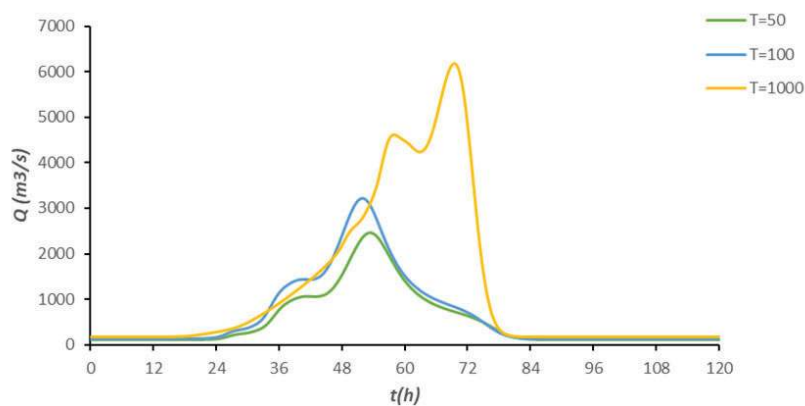
Πλημμυρογράφημα Εξόδου π. Καλαμά (μέσες συνθήκες)
