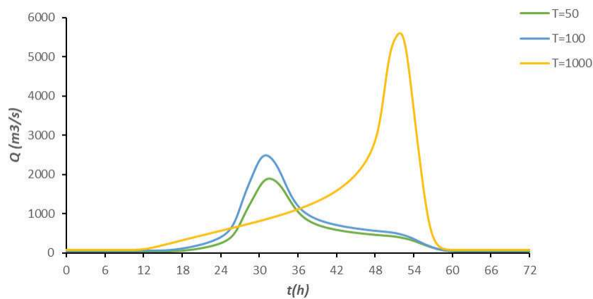
Πλημμυρογράφημα Εξόδου π. Αχέροντα (μέσες συνθήκες)
