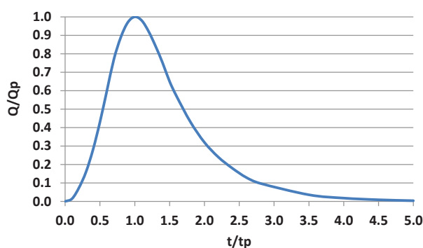
Εικόνα 3-18 Αδιαστατοποιημένο ΣΜΥ κατά SCS
