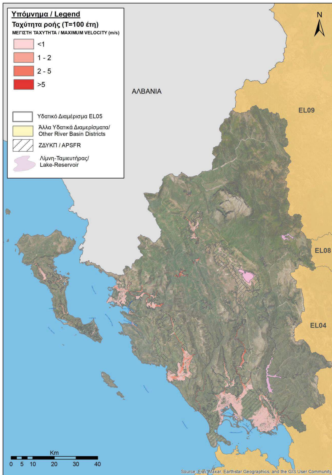
Εικόνα 3-49: Ταχύτητα ροής για πλημμύρα με περίοδο επαναφοράς T=100 έτη για το Υδατικό Διαμέρισμα Ηπείρου (EL05)
