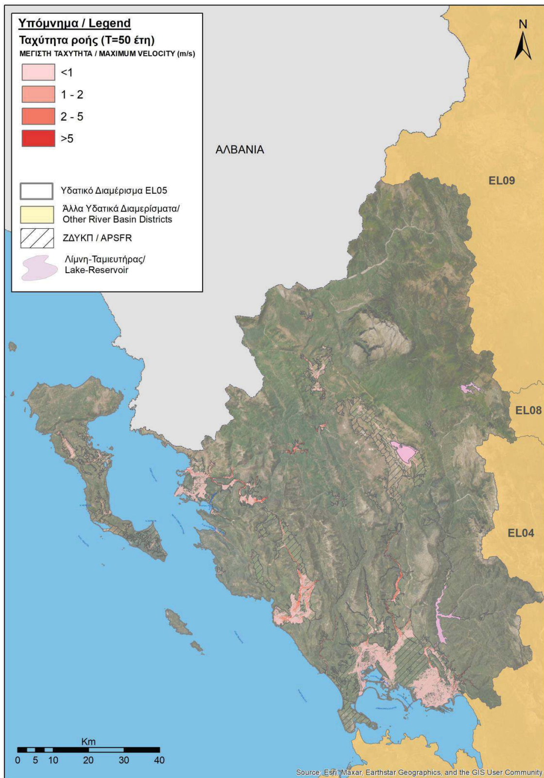
Εικόνα 3-48: Ταχύτητα ροής για πλημμύρα με περίοδο επαναφοράς T=50 έτη για το Υδατικό Διαμέρισμα Ηπείρου (EL05)
