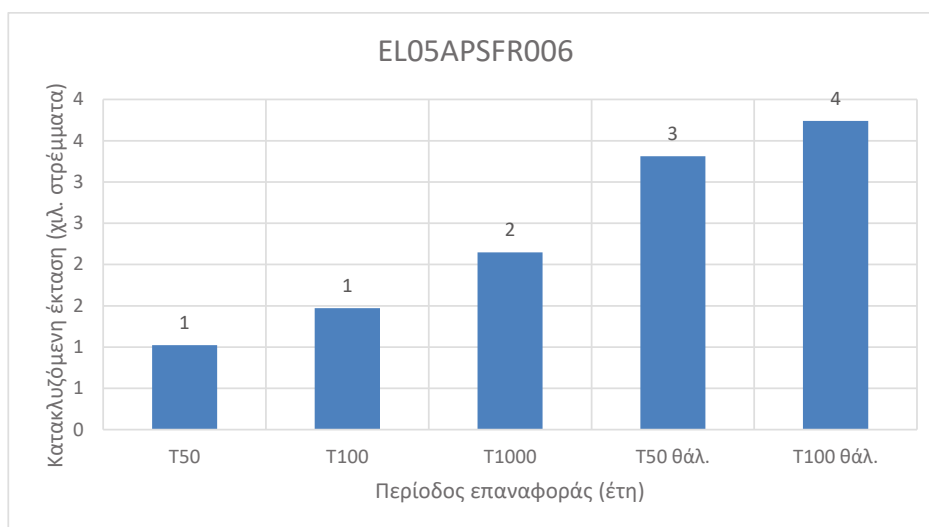
Εικόνα 3-28 Κατακλυζόμενες εκτάσεις για τις πλημμύρες περιόδου επαναφοράς 50, 100 και 1.000 ετών καθώς και για τις θαλάσσιες πλημμύρες περιόδου επαναφοράς 50 και 100 ετών στη EL05APSF006
