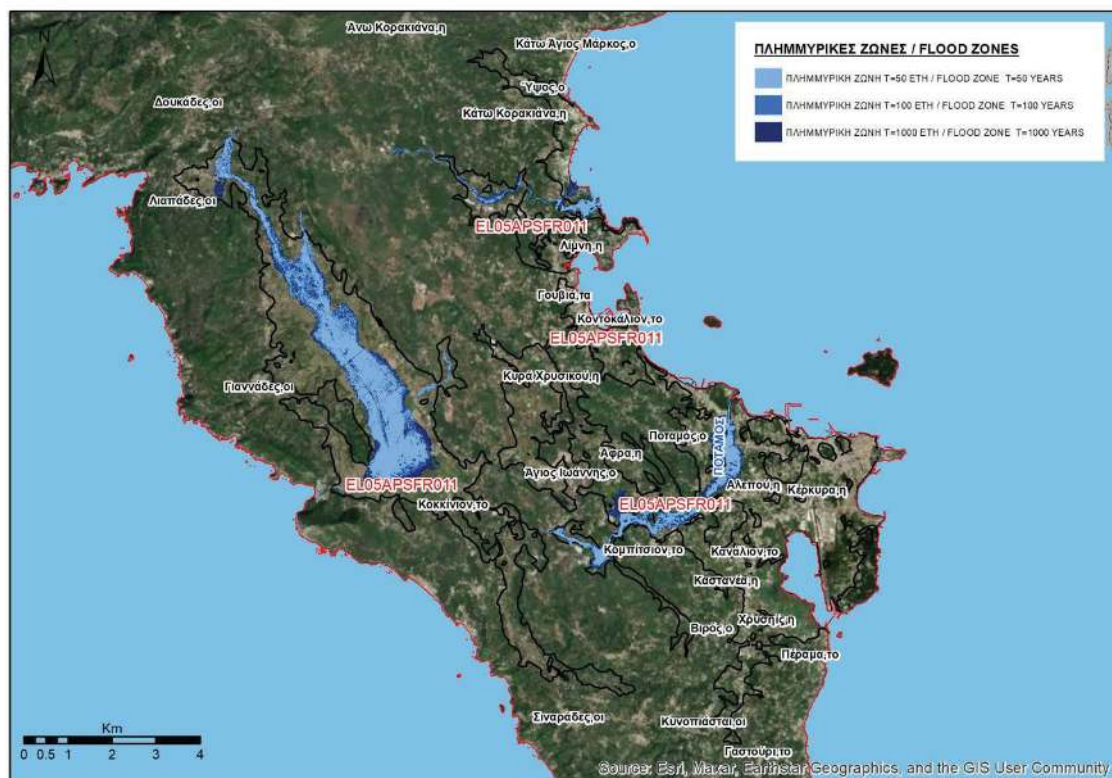
Εικόνα 3-39 Ζώνες κατάκλυσης για T=50, T=100 και T=1000 έτη για την EL05APSR011
