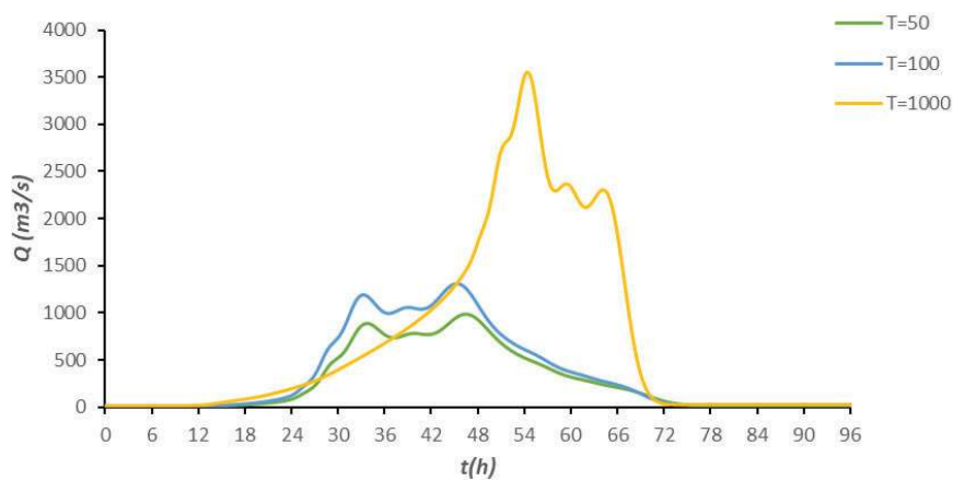
Πλημμυρογράφημα Εξόδου π. Λούρου (μέσες συνθήκες)
