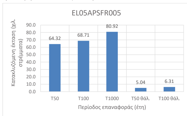
Εικόνα 3-26 Κατακλυζόμενες εκτάσεις για τις πλημμύρες περιόδου επαναφοράς 50, 100 και 1.000 ετών καθώς και για τις θαλάσσιες πλημμύρες περιόδου επαναφοράς 50 και 100 ετών στη EL05APSFR005
