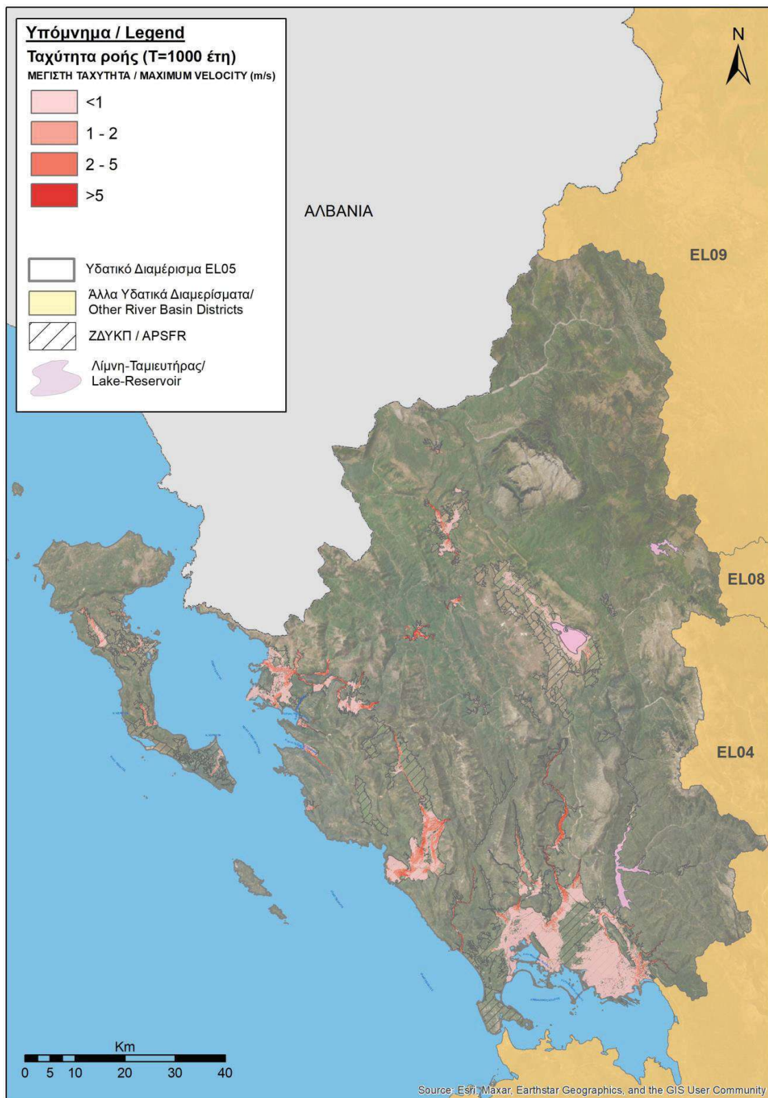
Εικόνα 3-50: Ταχύτητα ροής για πλημμύρα με περίοδο επαναφοράς T=1000 έτη για το Υδατικό Διαμέρισμα Ηπείρου (EL05)
