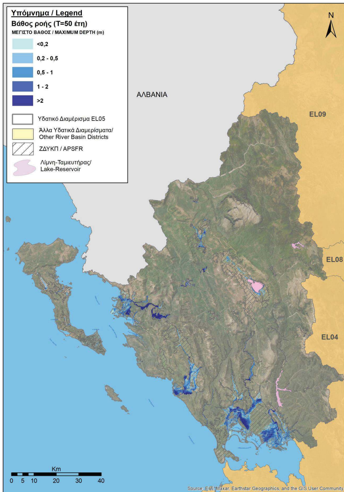
Εικόνα 3-45: Βάθος ροής και μέγιστο εύρος κατάκλυσης για πλημμύρα με περίοδο επαναφοράς T=50 έτη για το Υδατικό Διαμέρισμα Ηπείρου (EL05)
