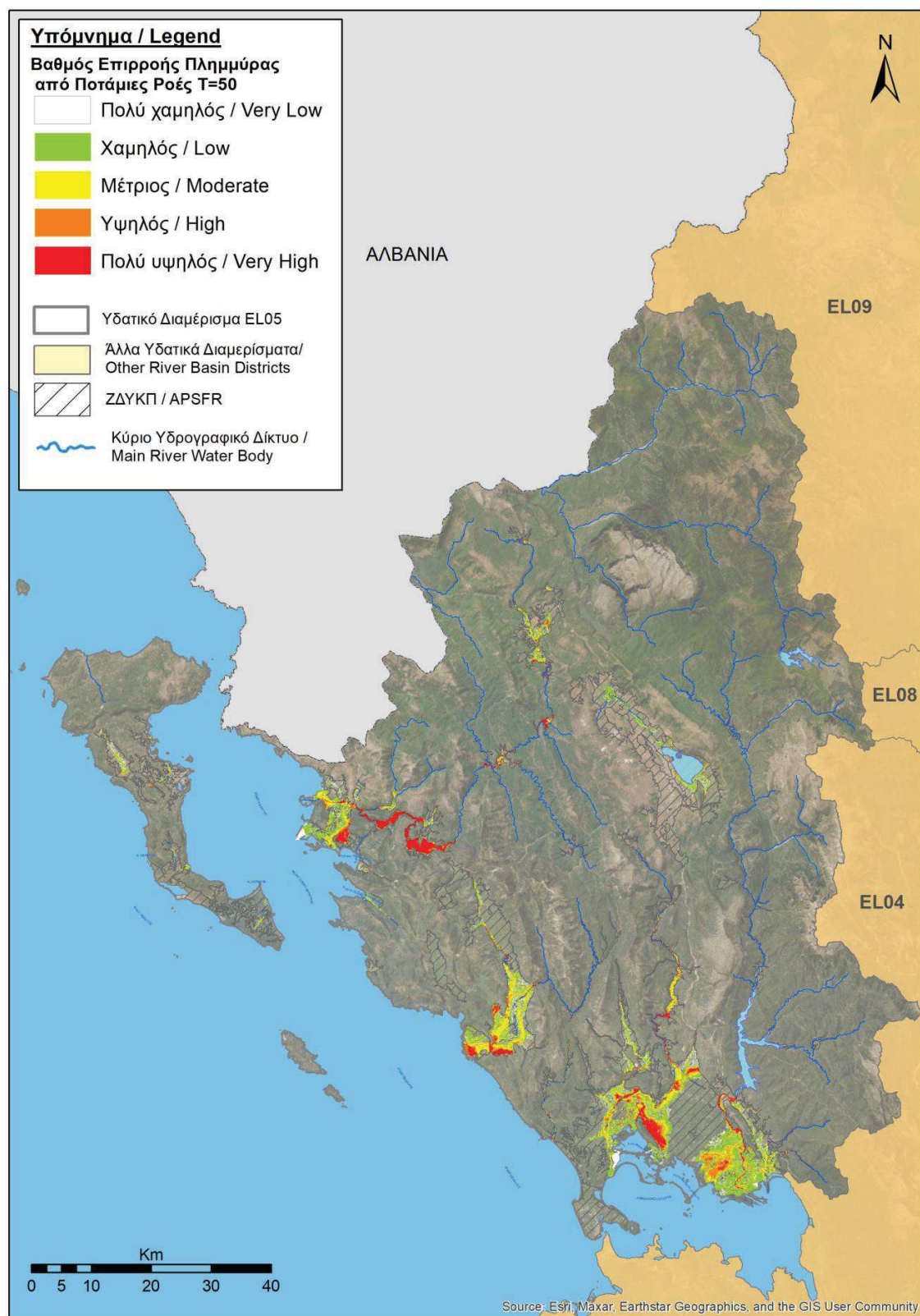
Εικόνα 3-100: Βαθμός επιρροής έντασης πλημμύρας (Αποτίμηση πλημμυρικής επικινδυνότητας – Flood Hazard) από ποτάμια [BA(T)] για T=50 έτη στο EL05
