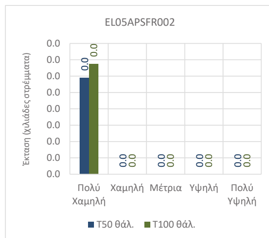
Εικόνα 3-72 Έκταση που αντιστοιχεί σε κάθε κατηγορία κινδύνου πλημμύρας, ανά περίοδο επαναφοράς για τη EL05APSFR002
