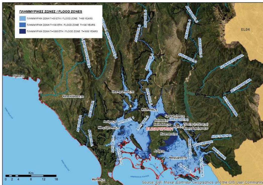
Εικόνα 3-22 Ζώνες κατάκλυσης για T=50 , T=100 και T=1000 έτη για την EL05APSF001
