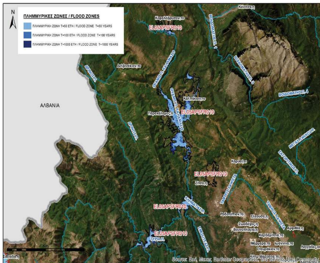
Εικόνα 3-37 Ζώνες κατάκλυσης για T=50, T=100 και T=1000 έτη για την EL05APSF010
