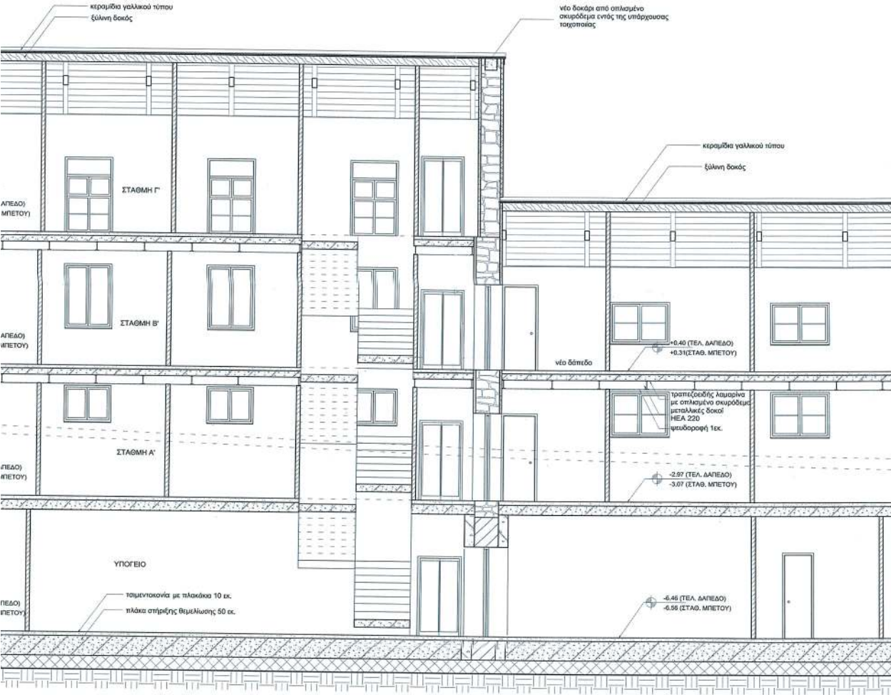
ΤΟΜΗ Α-Α ΚΛΙΜΑΚΑ 1:50
